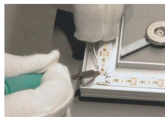
Zusammenführung LED-Flexbänder und Alu-Profile
