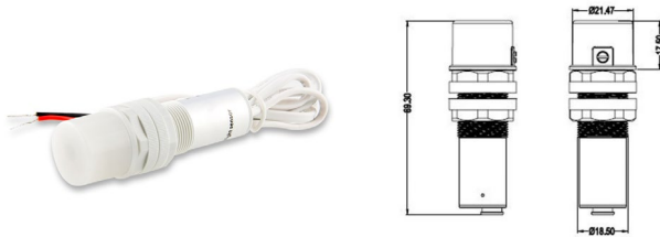
112619 | Tageslicht Sensor passiv zur Parallelschaltung in aktive 1-10V Steuersignalleitungen Kompatibel mit LED Multi Trafo 111989
