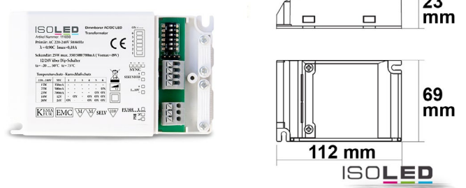
111989 | LED MULTI Trafo 12V/24V/350mA/500mA/700mA, Push + 1-10V dimmbar, SELV Kompatibel mit LED Tageslicht Sensor 112619
