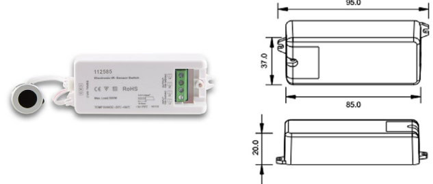
112585 | Wisch-Schalter mit Sensorkopf silber, Wischdistanz 6cm, 230V, 500VA
