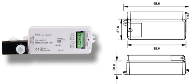
112587 | PIR Bewegungs-Sensor mit Sensorkopf, Erfassung max. 3m, 230V, 500VA
