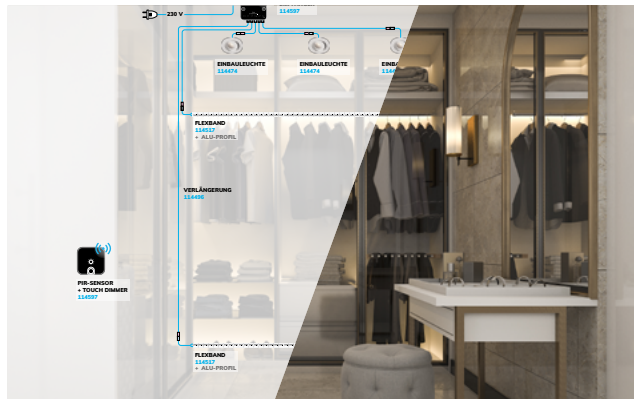
Armoire
