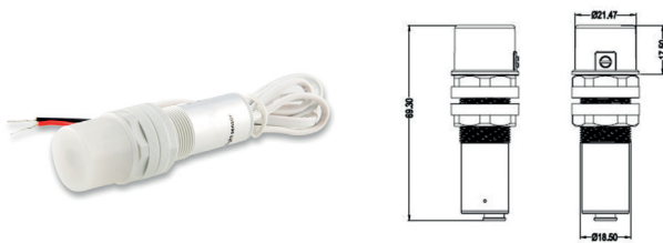
112619 | Capteur de lumière du jour passif pour une connexion parallèle dans les lignes de signaux de commande actives 1-10V Compatible avec le transformateur Multi LED 111989
