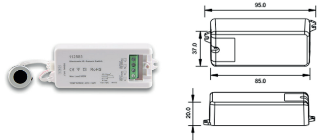
112585 | Interrupteur d'essuyage avec tête de détection argentée, distance d'essuyage 6cm, 230V, 500VA
