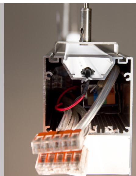
Profilé luminaire LED UP&DOWN1 (113483) avec suspension à fil et transformateur SYS-ONE (113521) intégré et antenne led out.
